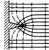
Abb. 28. Kraftlinien und Niveaulinien bei einer leitenden Spitze.
